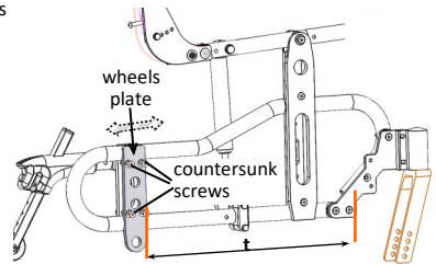
pic.12.3: Displacement of the posterior wheels
