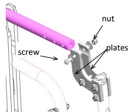
fig. 11.2: Anterior part depth adjustment
