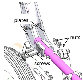
fig. 11.1: Posterior part depth adjustment
